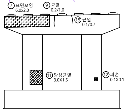
A2 방향
