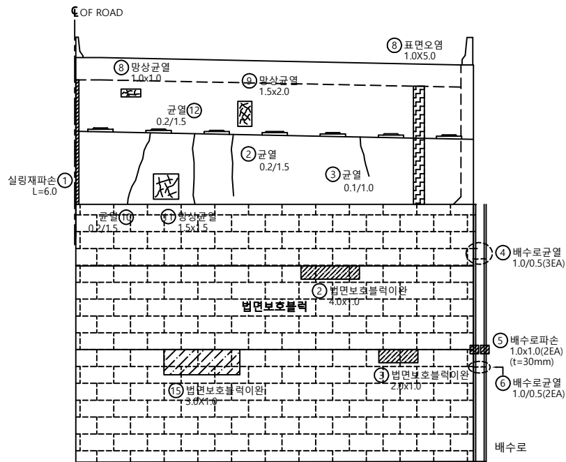
정면도
