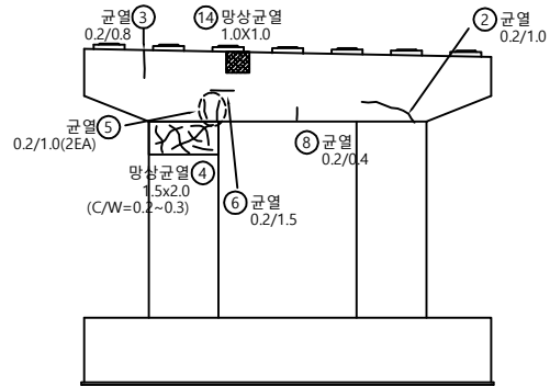
A1 방향
